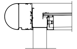
Optionale Runde Rinnenkappe
