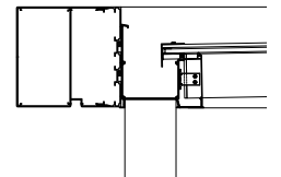
Optionale Gerade Rinnenkappe
