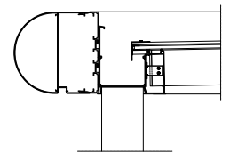
Optionale Runde Rinnenkappe
