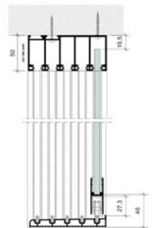
Verstellbare Rollen im höchsten Position
