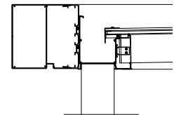
Optionale Gerade Rinnenkappe
