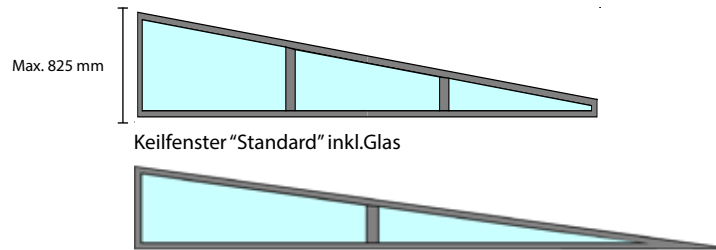
Keilfenster "auf Null" inkl. Glas (unter 4° nicht möglich)
